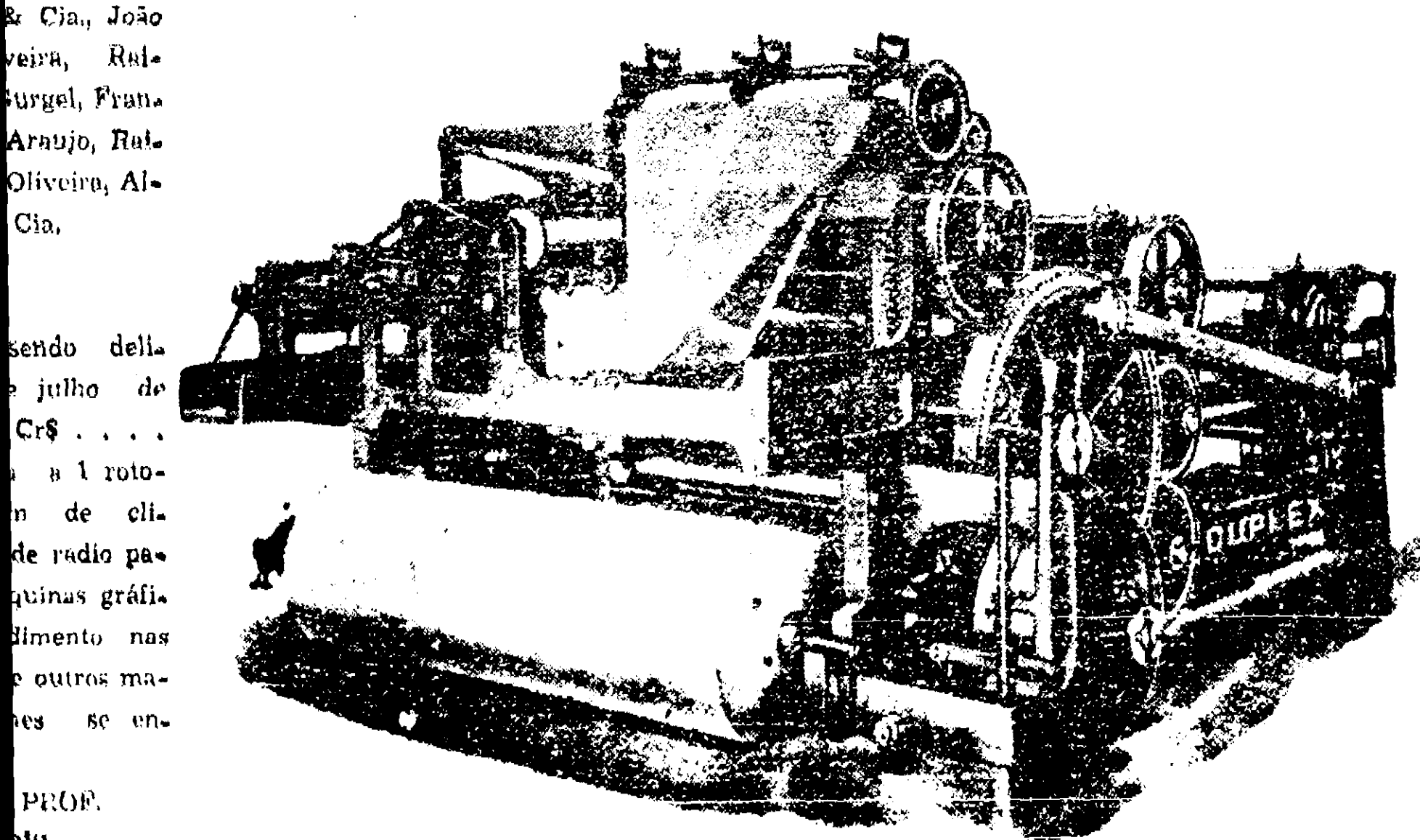
OUTRA PERSPECTIVA DA ROTOPLANA DUPLEX
