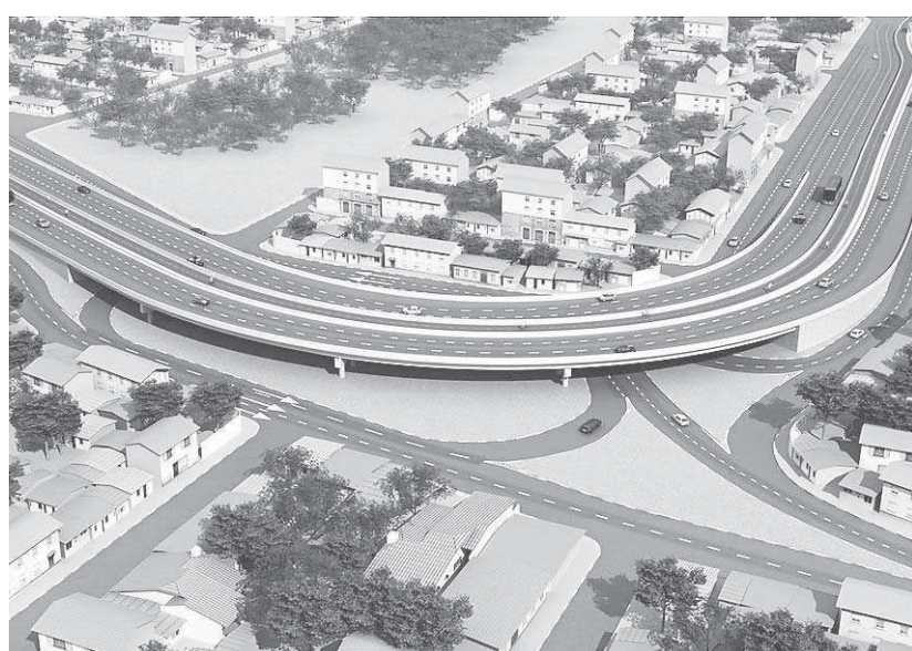
► Complexo viário da Urbana inclui obras também nas avenidas Felizardo Moura e Capitão-Mor Gouveia, que deve ganhar um viaduto em seu final
